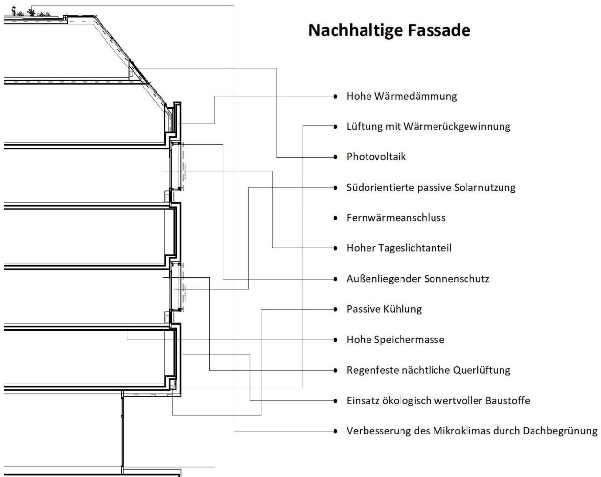
Abbildung 7: Integration von Gebäudetechnik mit horizontaler und vertikaler Verteilung innerhalb der Fassade
